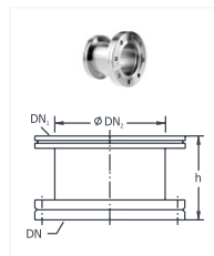
Адаптеры ISO-CF / K для CBB соединений Материал исполнения: нержавеющая сталь
