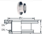
Редукторы ISO-K / K
