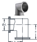
Уголки под 90 градусов сварные
