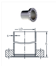
Фланцы с патрубком не вращающийся Материал исполнения: нержавеющая сталь
